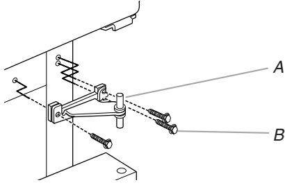
A. Bisagra central B. Tornillos de cabeza hexagonal para bisagra de 5/16"
