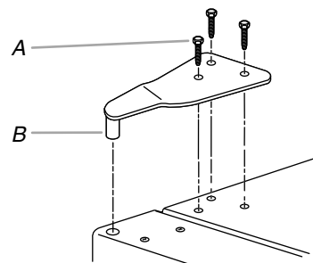
A. Tornillos de cabeza hexagonal para bisagra de 5/16" B. Pasador de la bisagra superior
